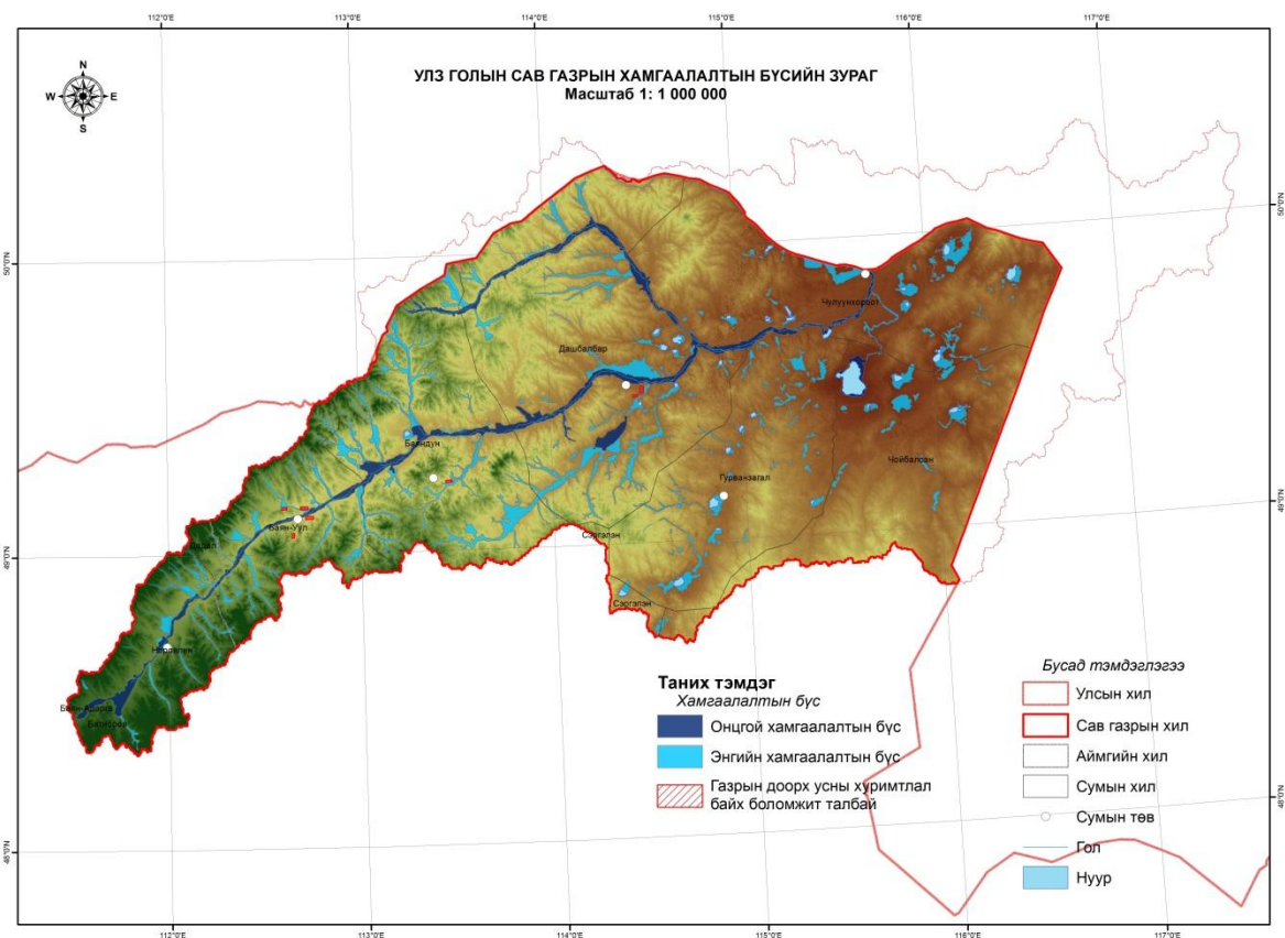
Зураг. Улз голын сав газрын усан сан бүхий газар, усны эх үүсвэрийн онцгой болон энгийн хамгаалалтын бүсийн зураг
