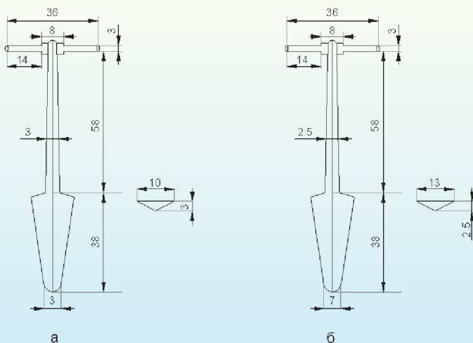
5 дугаар зураг. Мөчир суулгагч Колесовын царил
