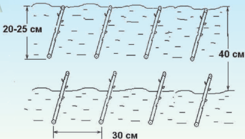
4 дүгээр зураг. Мөчир суулгах бүдүүвч
