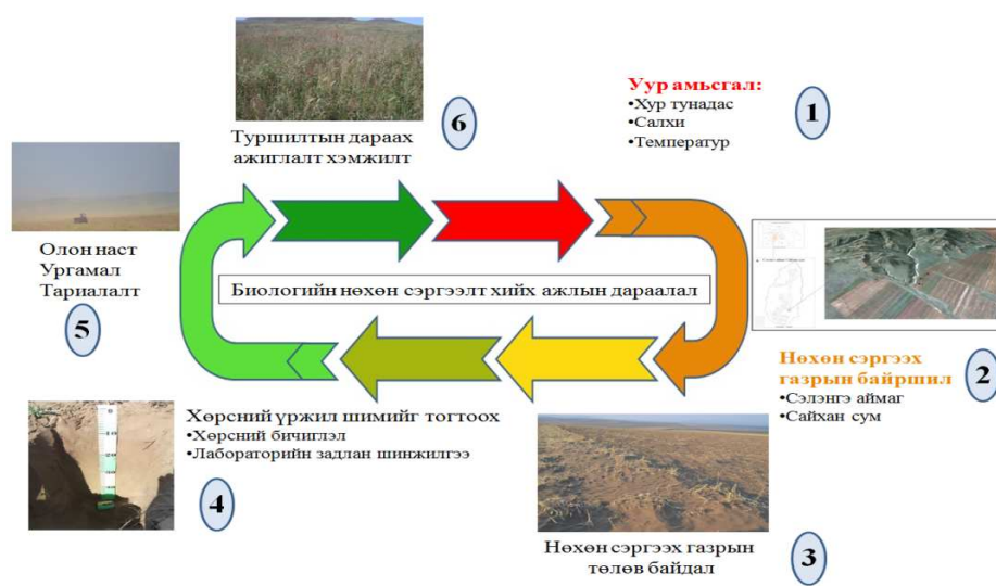
Зураг 13. Тариалангийн нөлөөгөөр эвдэрсэн газрыг биологийн аргаар нөхөн сэргээх ажлын бүдүүвч
