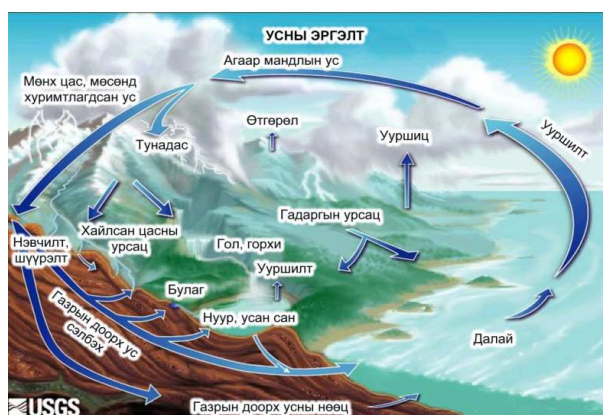
Зураг 15. Дэлхийн усны эргэлтийн зураг.
