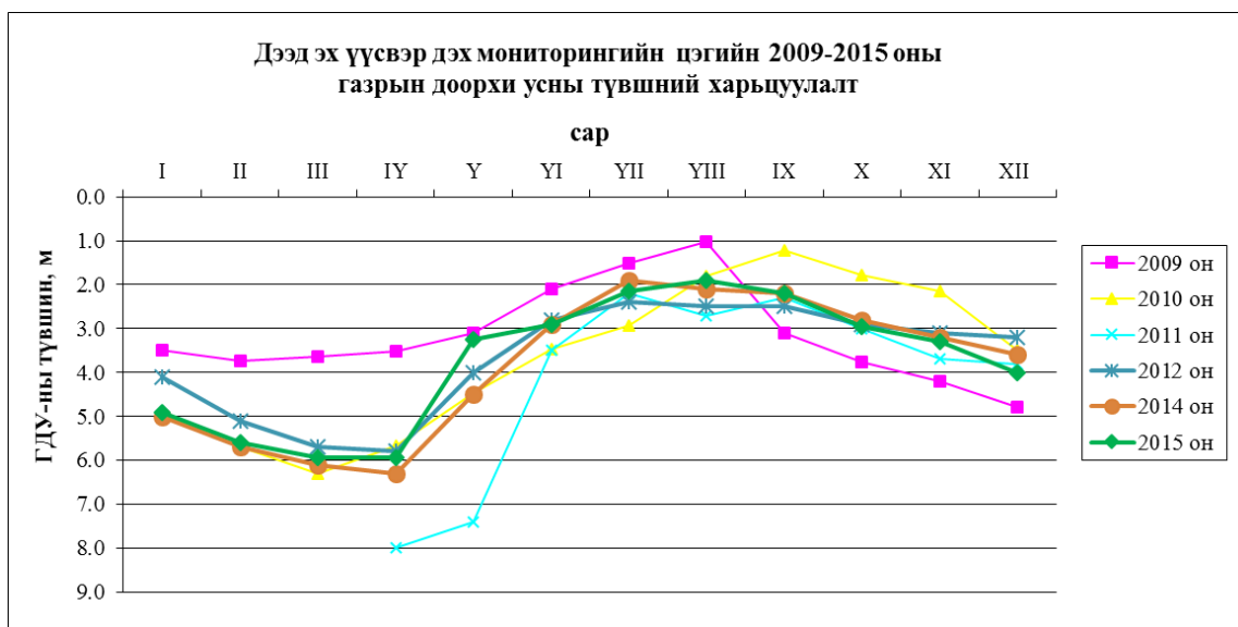
3 дугаар тахирмаг. Мониторингийн 2р цэгийн олон жилийн түвшний харьцуулалт
