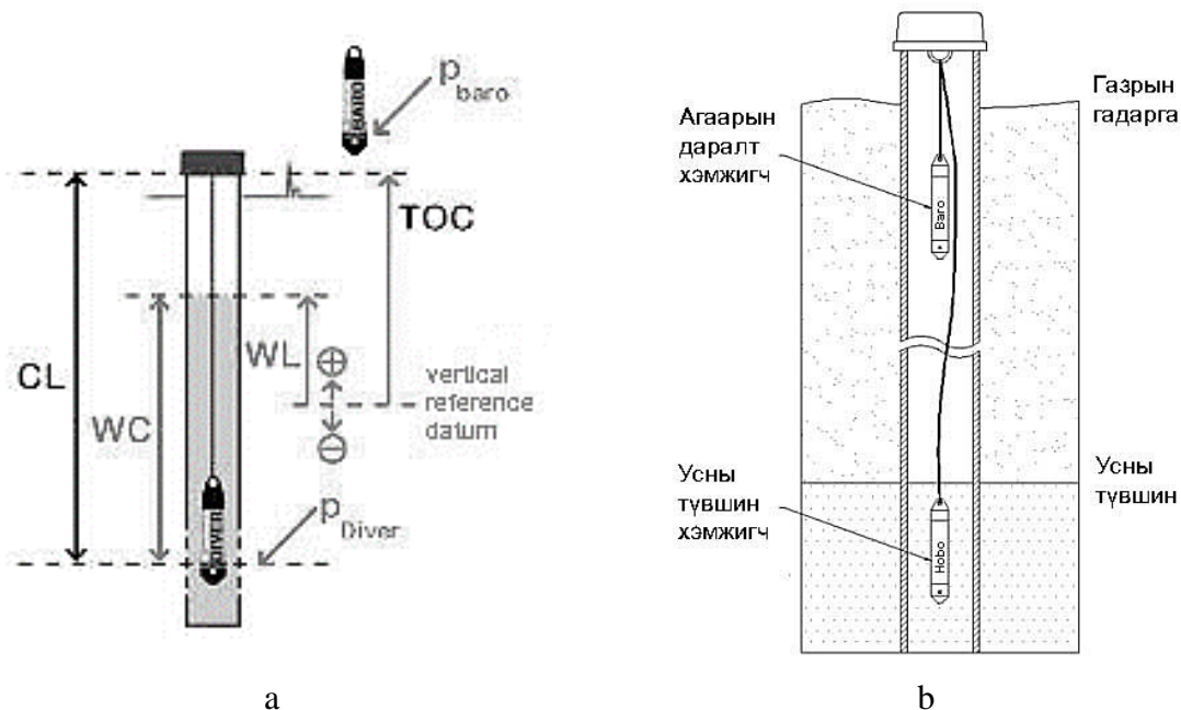
2 дугаар зураг. a -Diver болон Baro, b -Hobo багаж суурилуулалт
