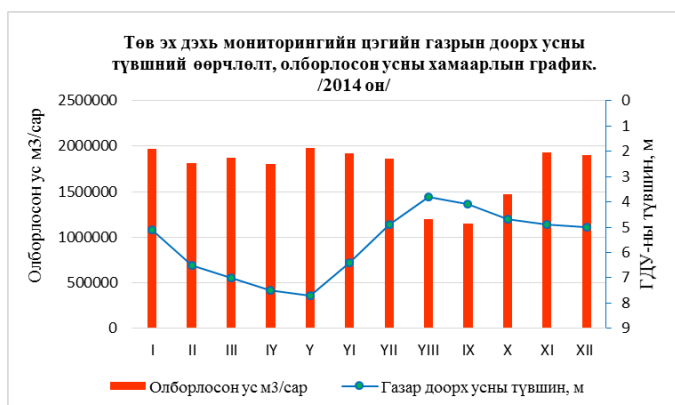
4 дүгээр тахирмаг. Мониторингийн 3р цэгийн усны түвшинг, олборлолттой харьцуулсан байдал
