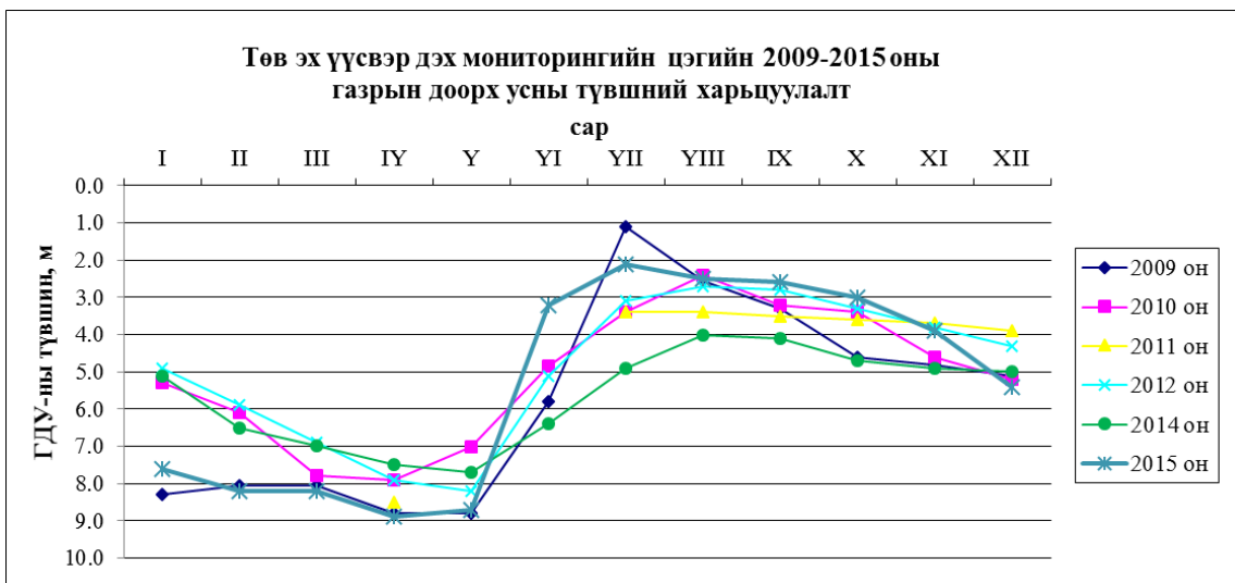
6 дугаар тахирмаг. Мониторингийн 3р цэгийн олон жилийн түвшний харьцуулалт
