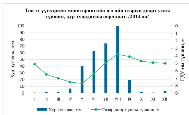
5 дугаар тахирмаг. Мониторингийн 3р цэгийн усны түвшинг, хур тунадастай харьцуулсан байдал
