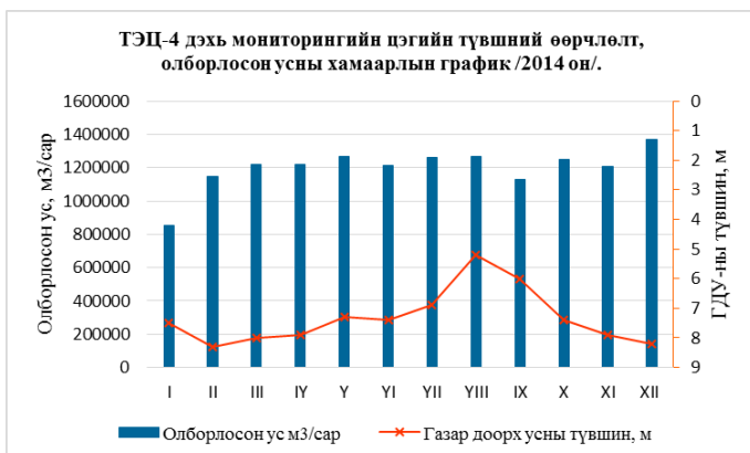
7 дугаар тахирмаг. Мониторингийн 8р цэгийн усны түвшинг, олборлолттой харьцуулсан байдал
